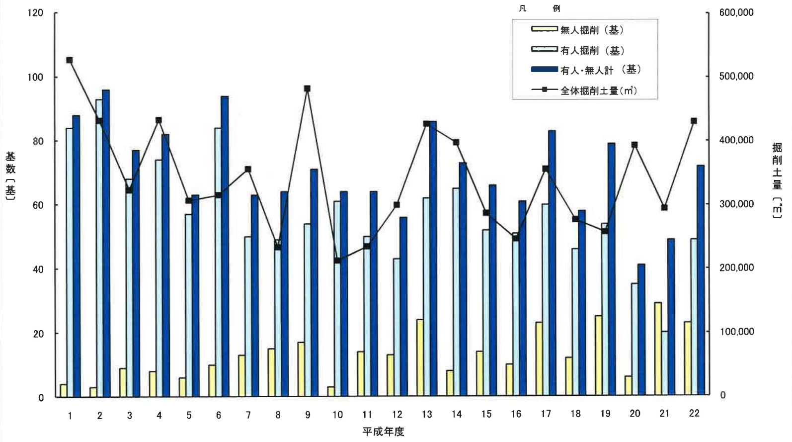
ニューマチックケーソン年度毎実績表
